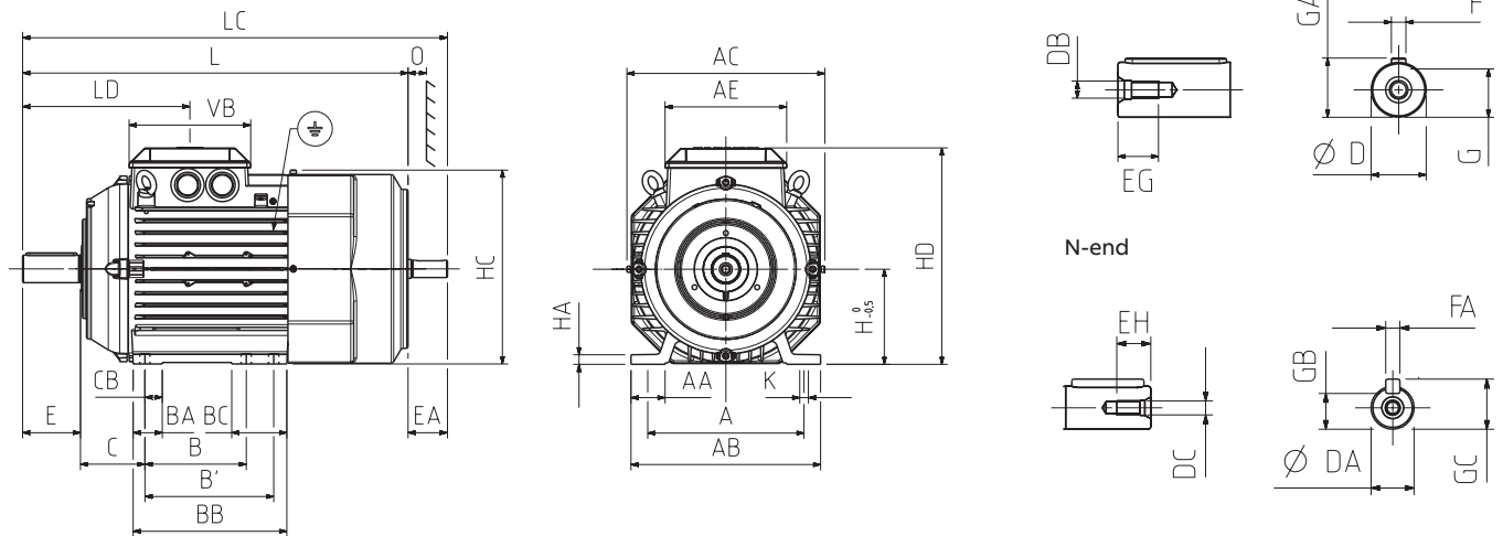
Mounting options IM B3 (IM 1001), IM B6 (IM 1051), IM B7 (IM 1061), IM B8 (IM 1071), IM V5 (IM 1011), IM V6 (IM 1031)
