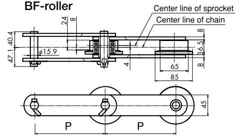
BF-roller
